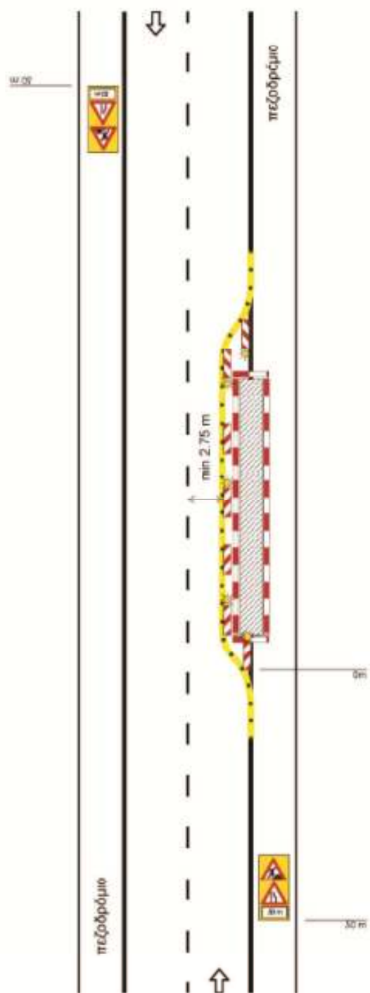
Σχέδιο 3.1.1 : Στένωση λωρίδας.
