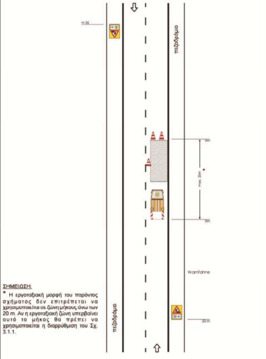
Σχέδιο 3.2.1 : Αποκλεισμός λωρίδας σε κύρια αστική οδό.
