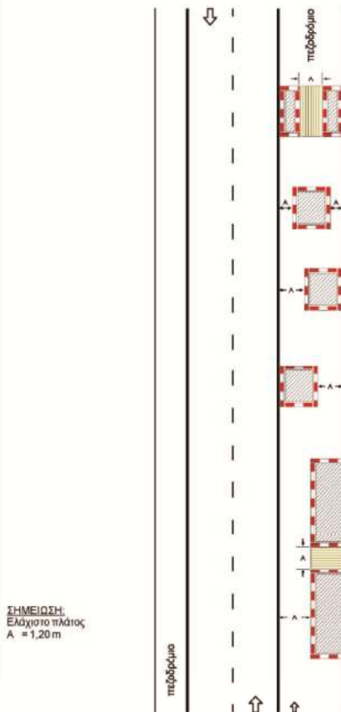
Σχέδιο 3.1.5 : Εργοτάξιο επί του πεζοδρομίου.
