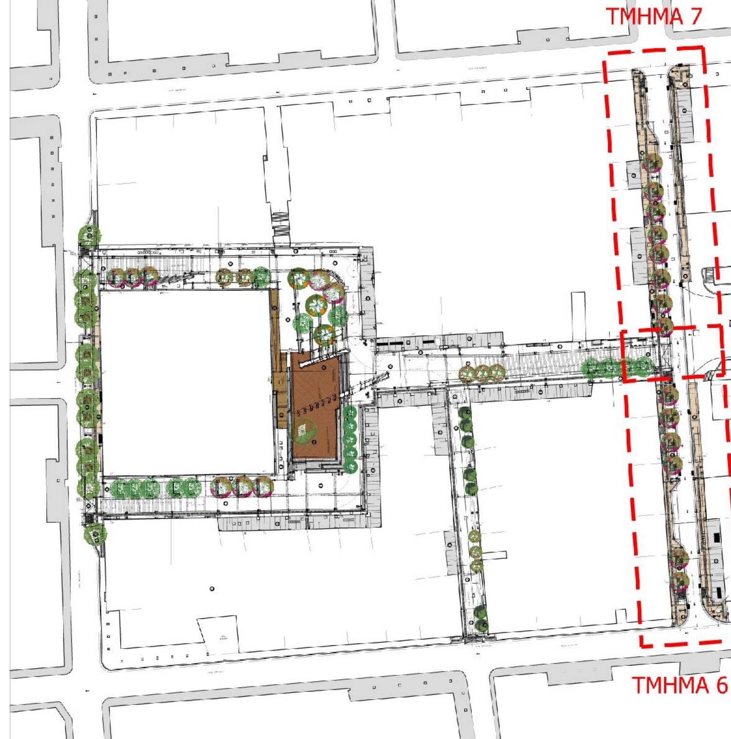
ΟΡΙΖΟΝΤΙΟΓΡΑΦΙΑ ΤΜΗΜΑ 7
